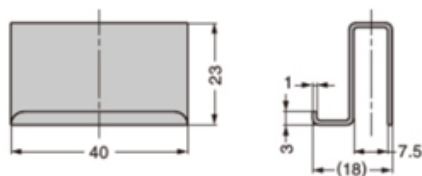
■寸法図
