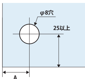
【ガラス加工図】
