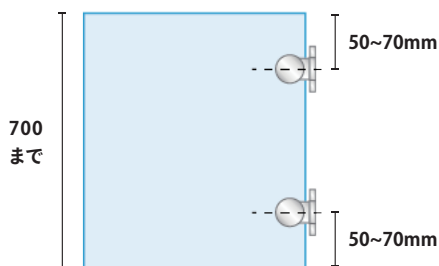
【ガラス加工図】
