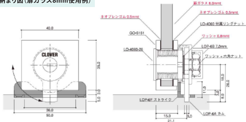
納まり図 (扉ガラス8mm使用例)
