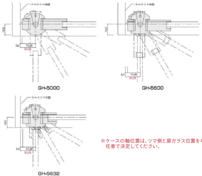
■軸位置、ツマ、扉ガラス関連寸法図
