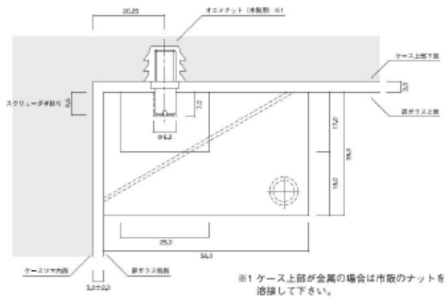
■上部スクリーダボ納まり寸法図
